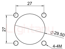
开孔尺寸
